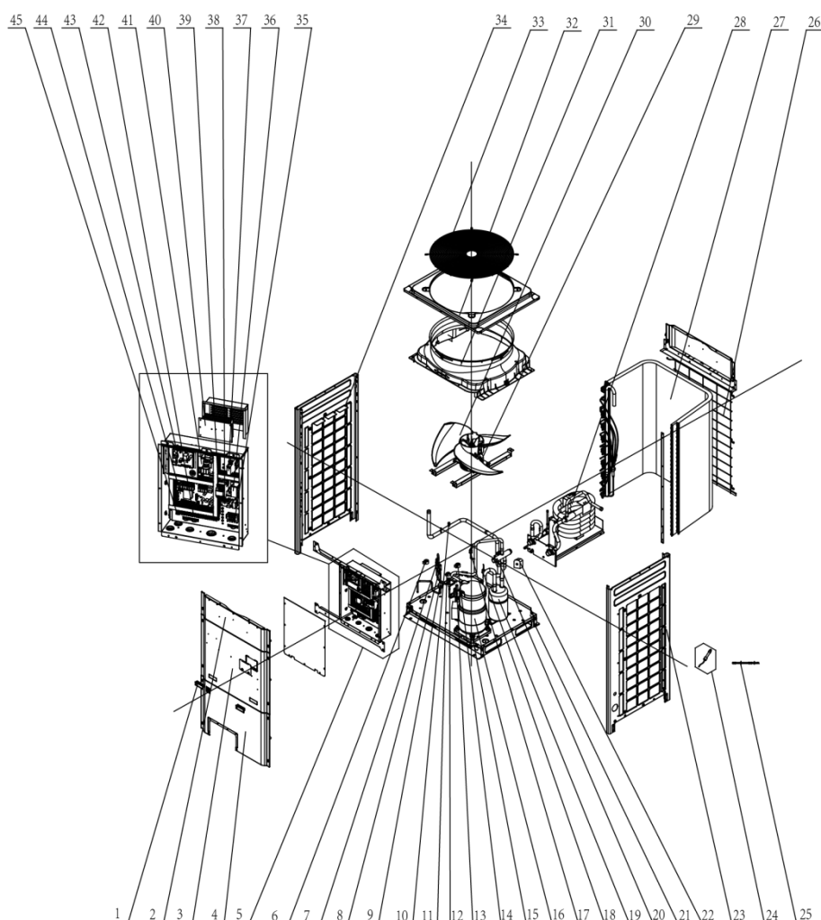
Список деталей CH-HP20CMNFM1:
