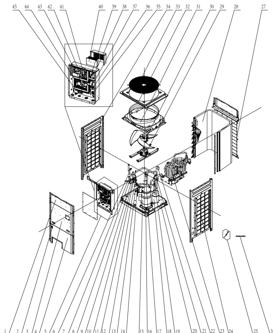
Список деталей CH-HP30CMNFM1:
