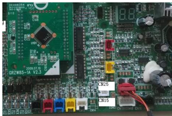
Рисунок подключения проводки главной платы
