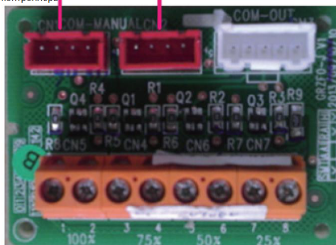
Рисунок подключения клем уровня жидкости
