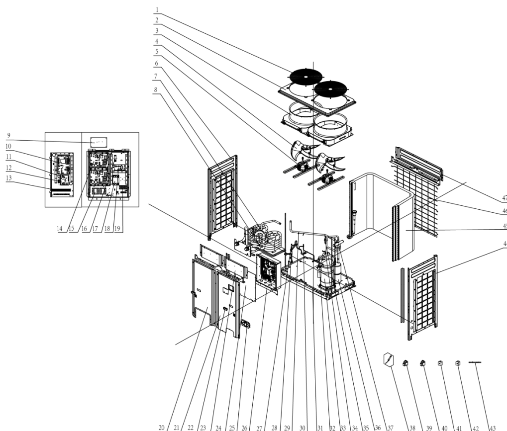
Список деталей CH-HP40CMNFM1:
