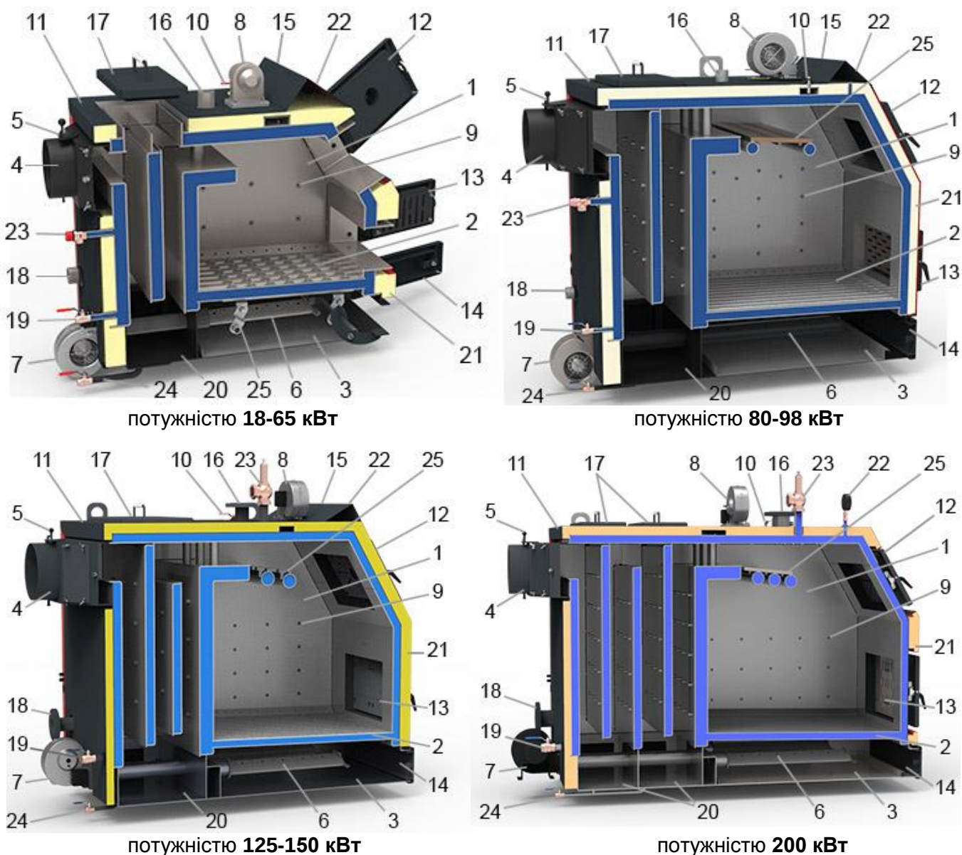
Рис.2 Будова котлів модельного ряду «Retra-3М»
